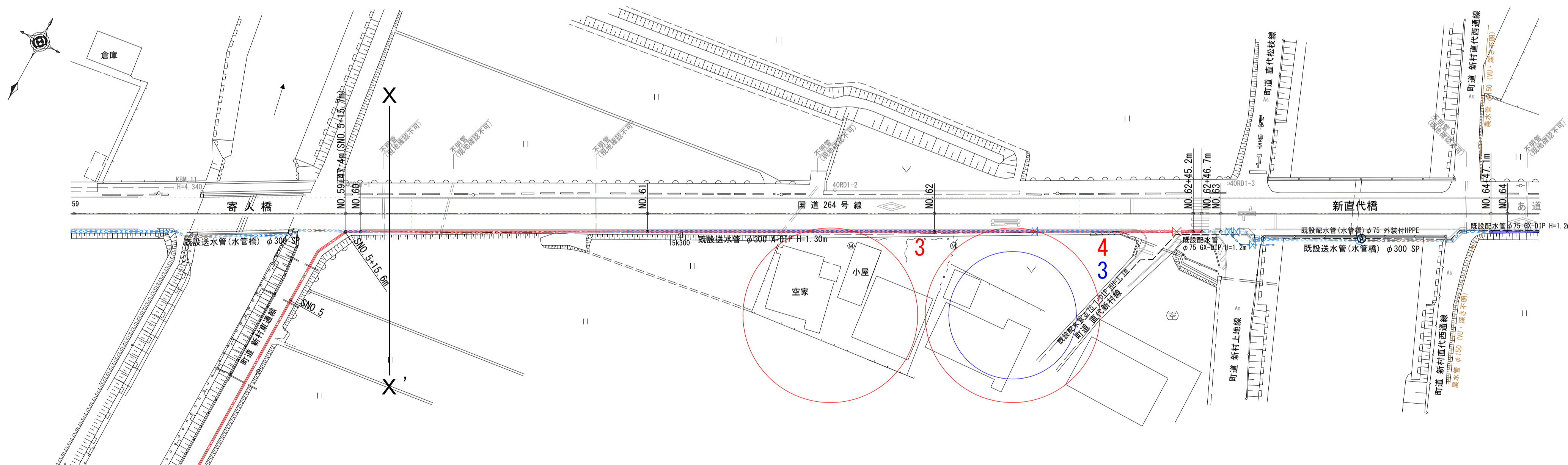
平面図 (2) S=1/500
