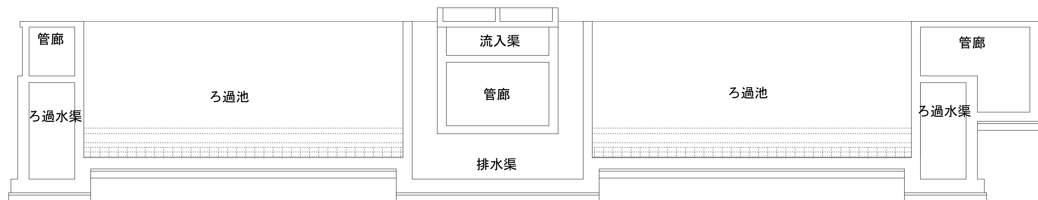
C-C' 断面
