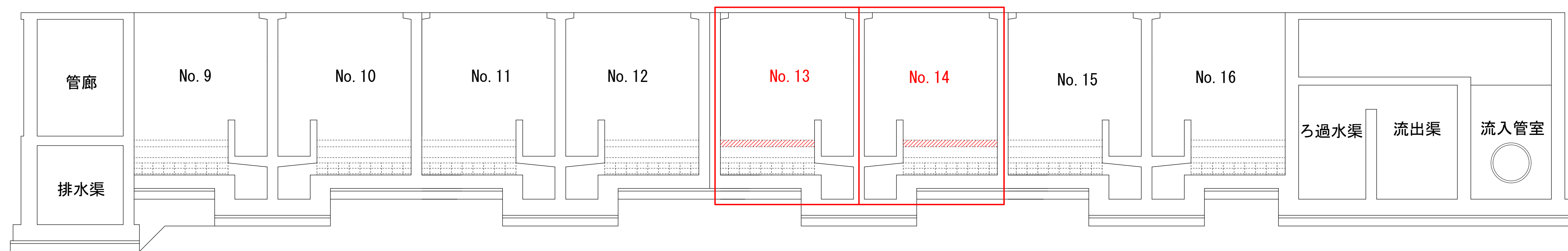
A-A' 断面
