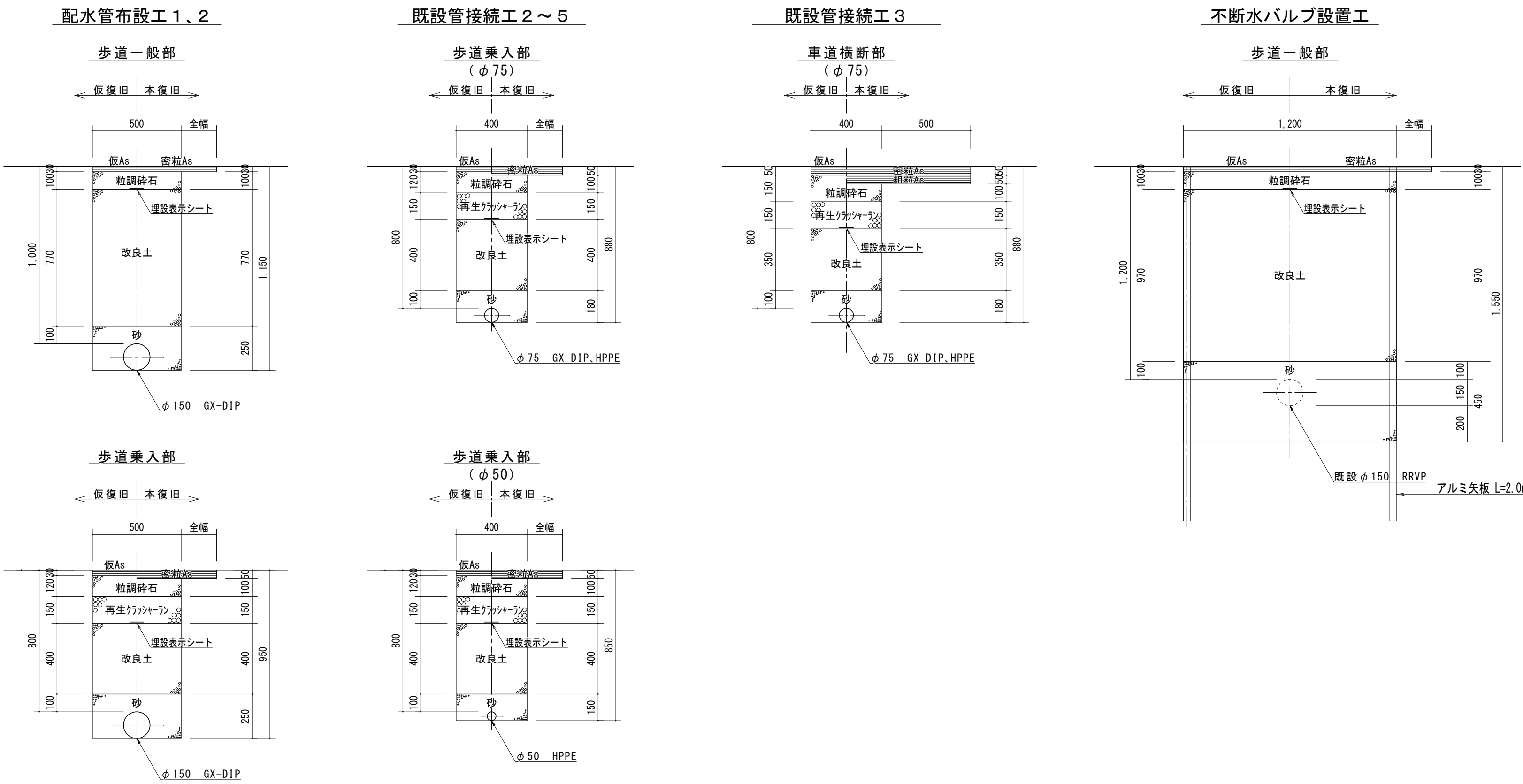
道路掘削復旧断面図 S=1/20
