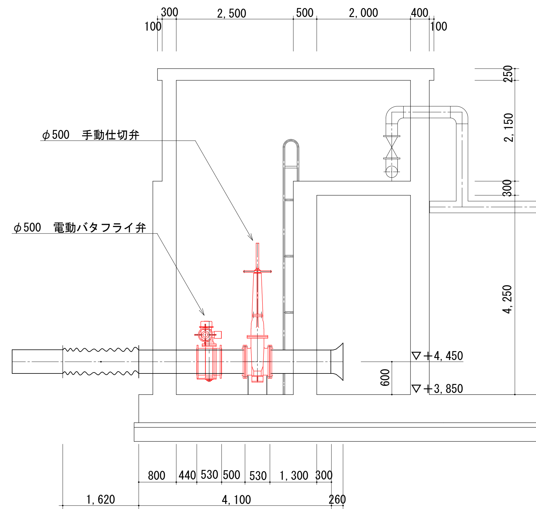
【B-B' 断面図】 更新設置後
