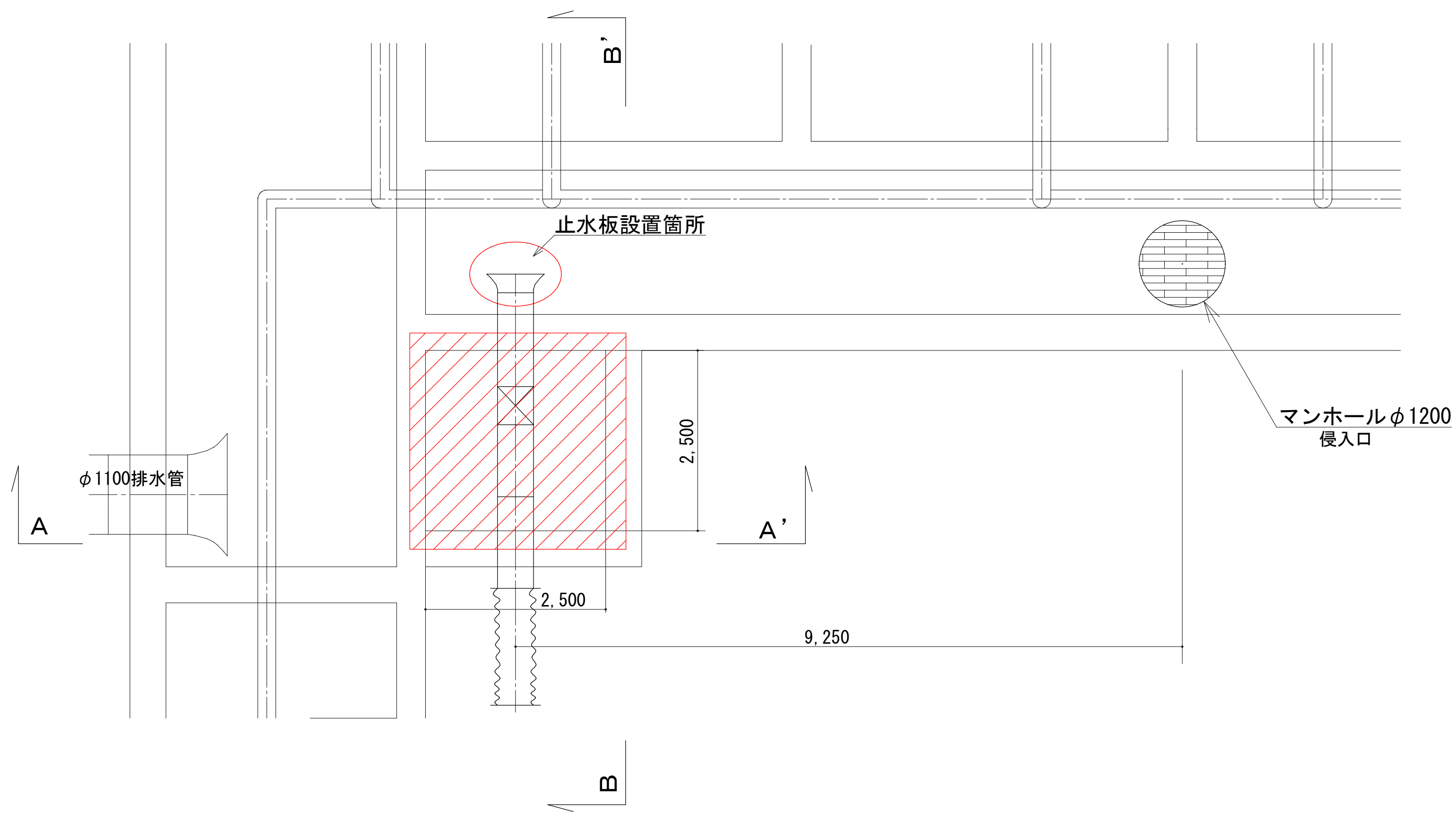
平面詳細図
