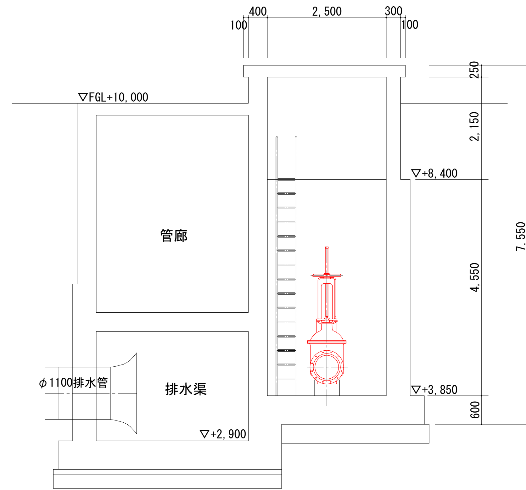
【A-A' 断面図】
