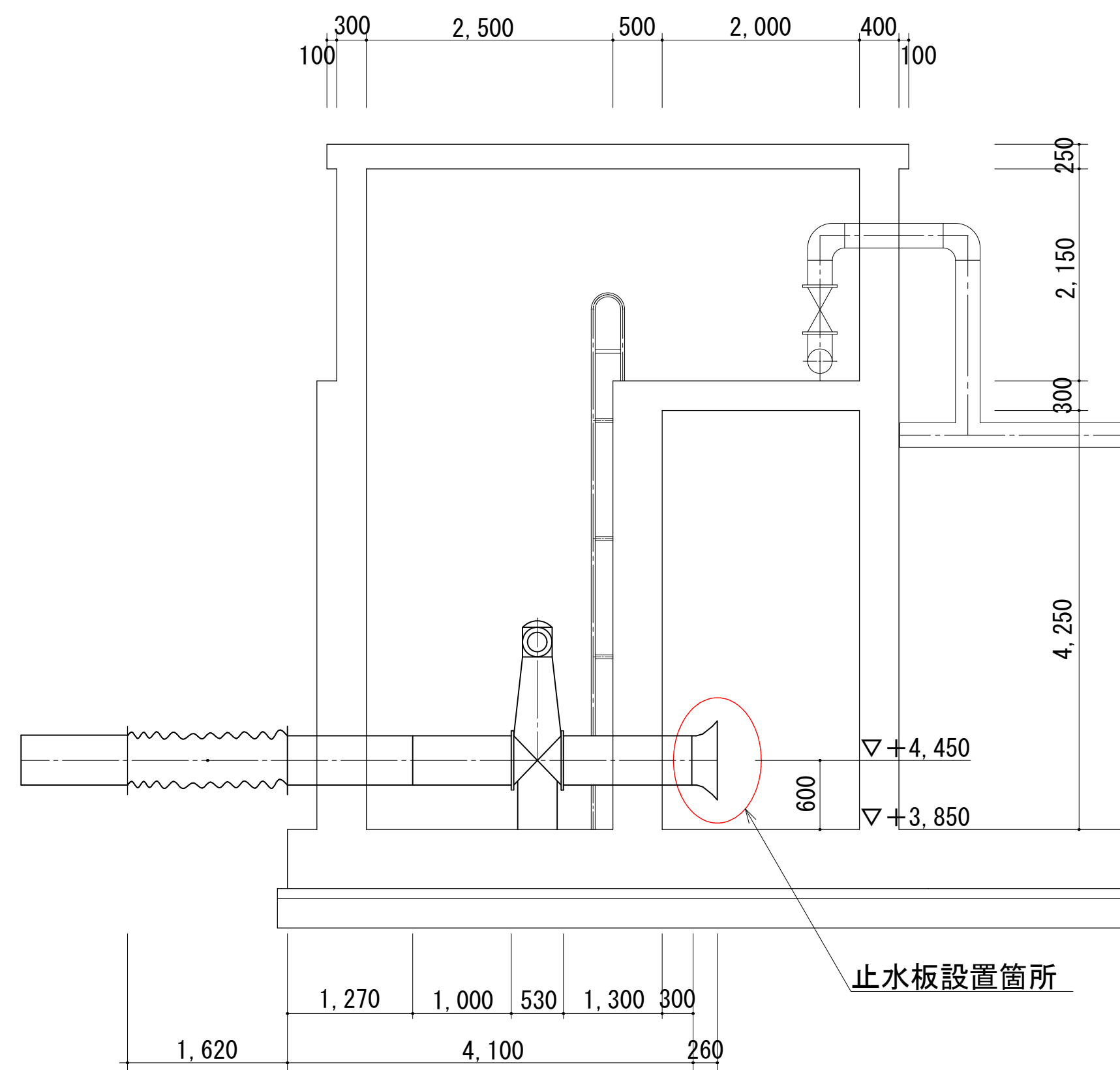
【B-B' 断面図】 現行
