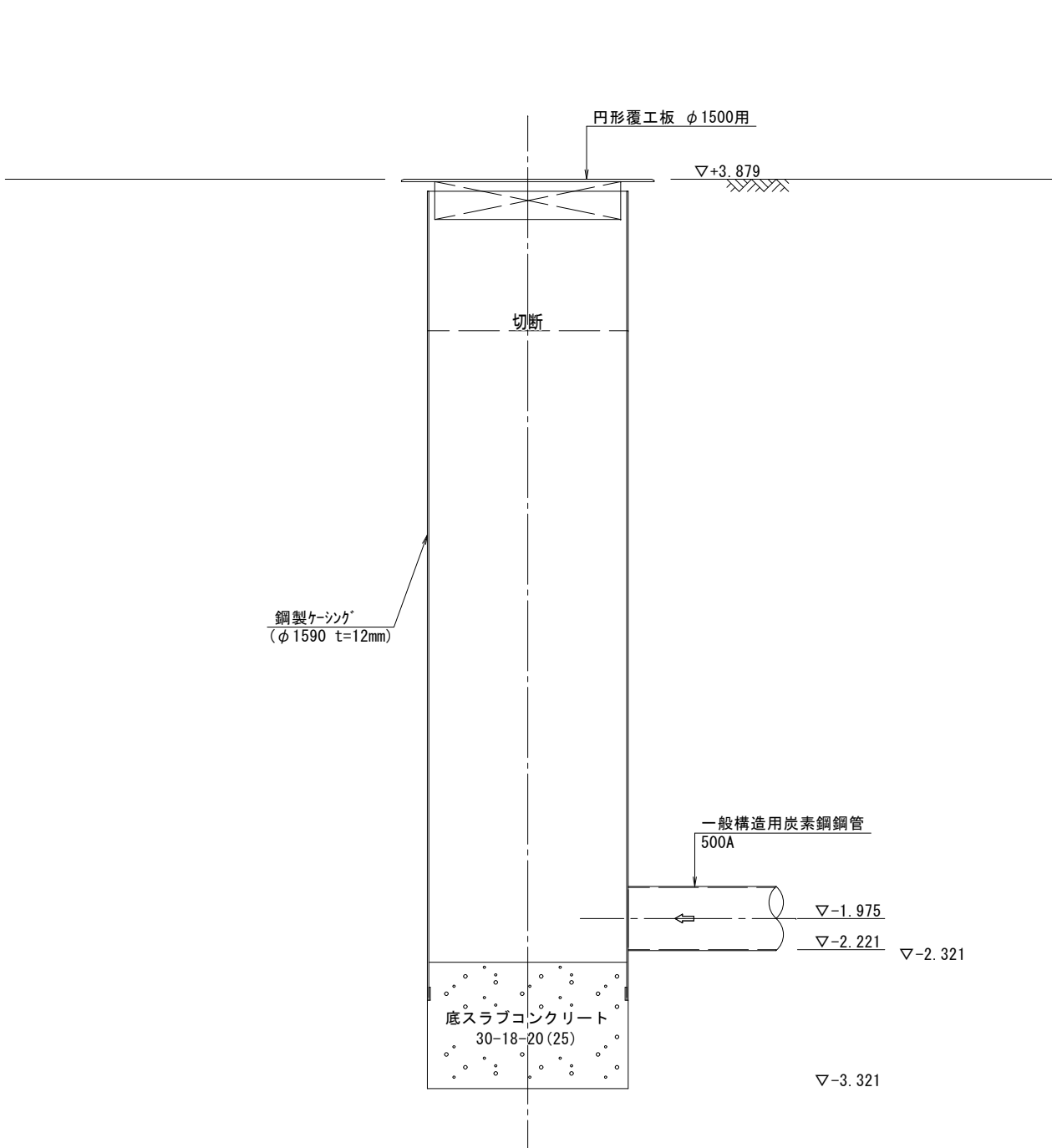
A-A 断面図 (底盤コンクリート打設・引抜完了図)
