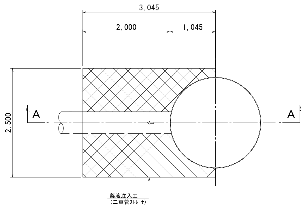
平面図
