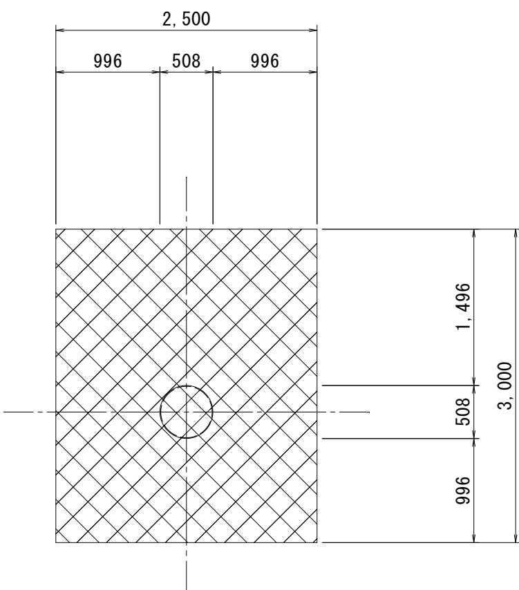
側面図
