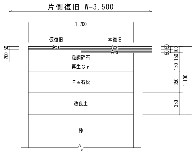
道路掘削復旧断面図 S=1/30
