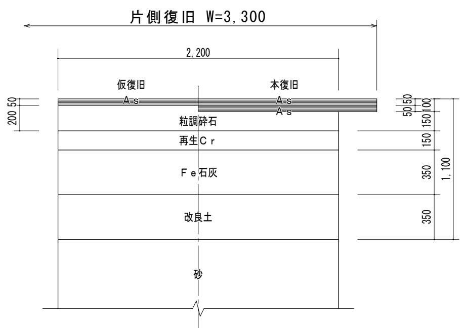
道路掘削復旧断面図 S=1/30
