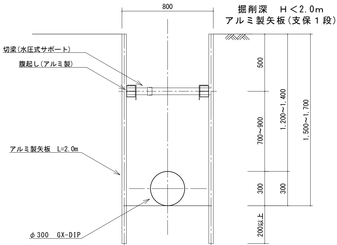
矢板設置標準図 S=1/20
