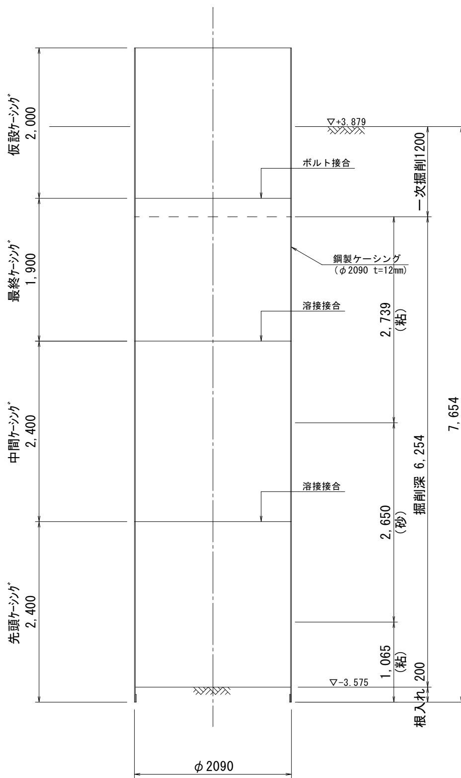
A-A断面図 (圧入掘削完了図)
