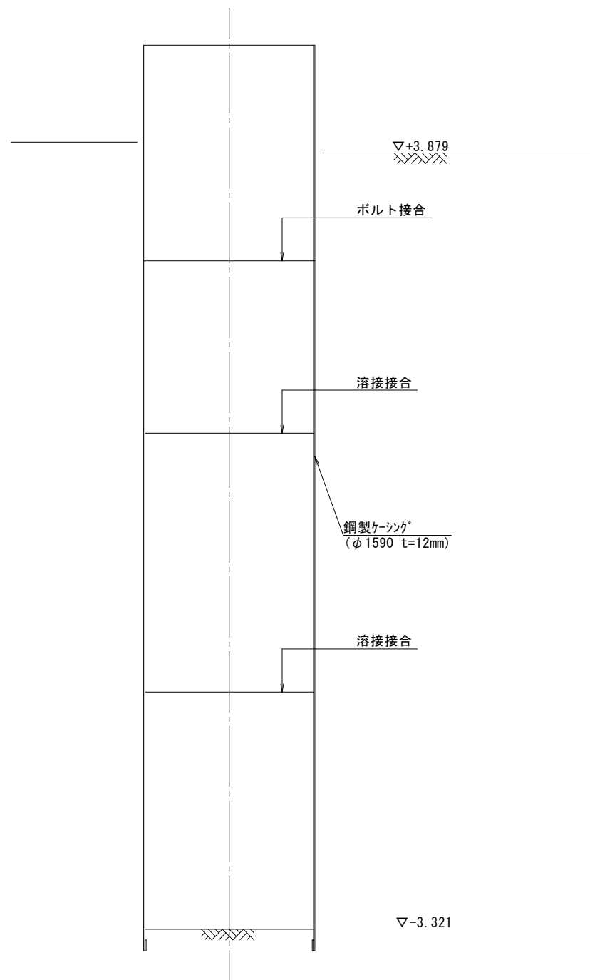
A-A 断面図 (圧入掘削完了図)
