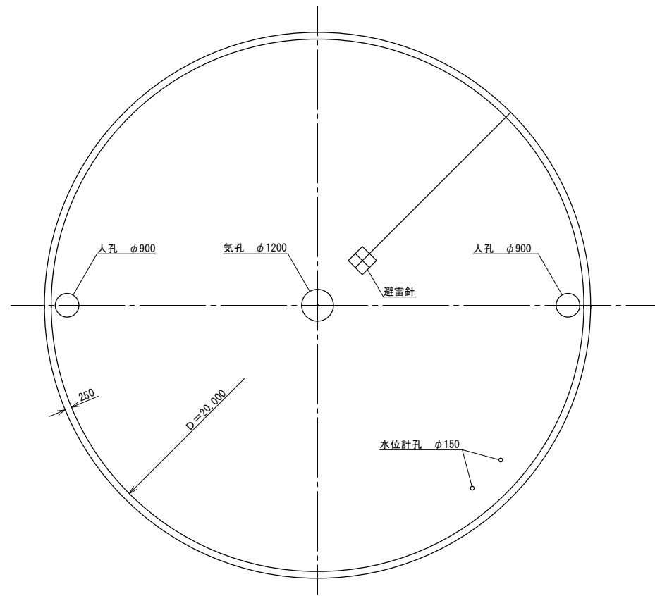
平面図
