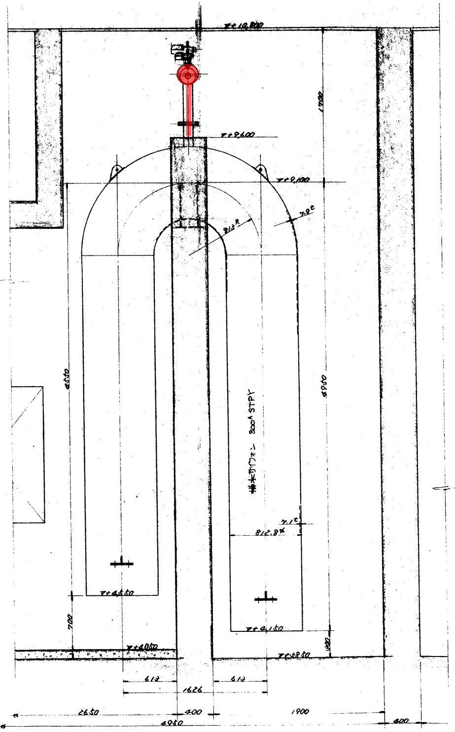
B-B 断面図
