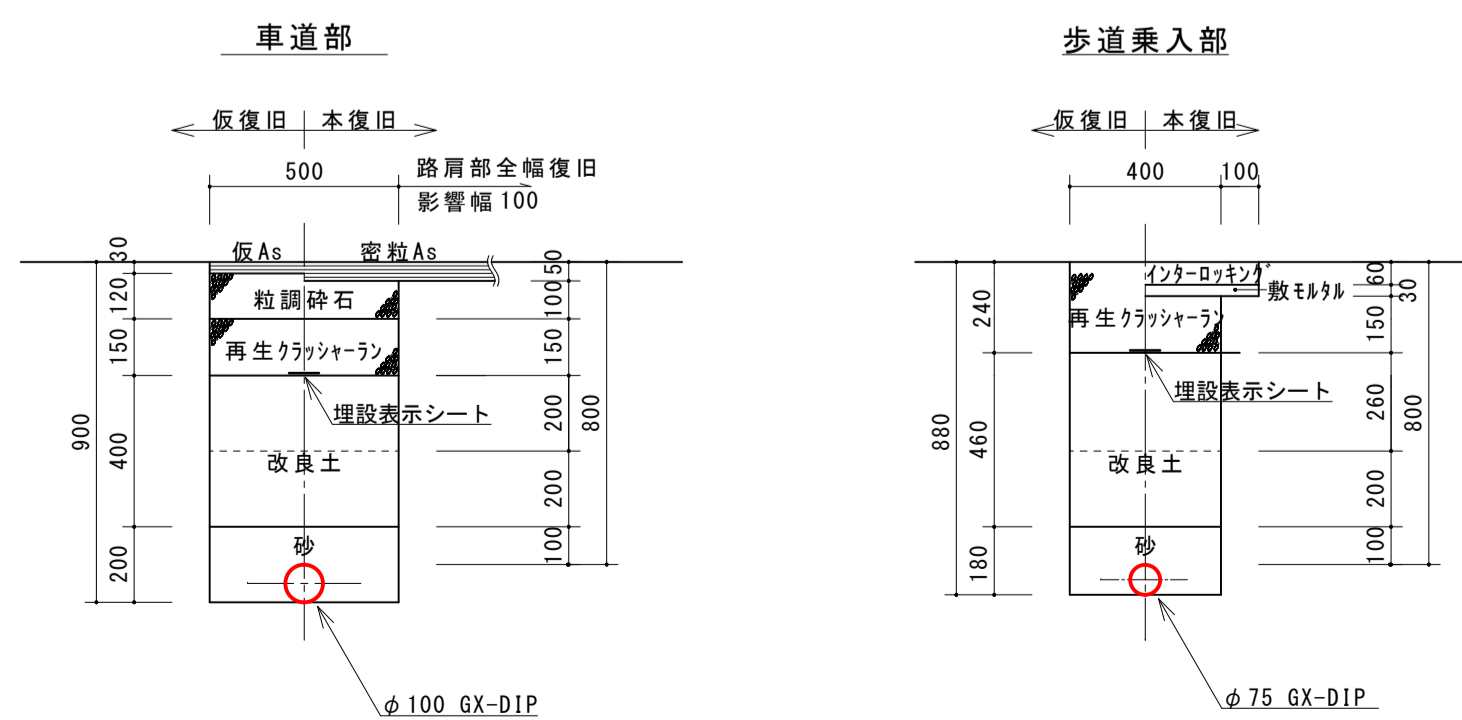
道路掘削復旧断面図 S=1/20
