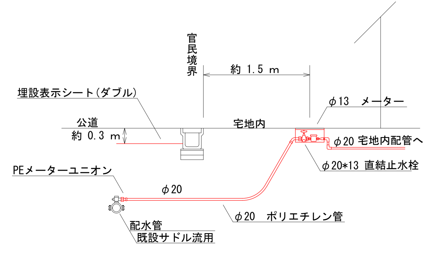
給水管標準図
