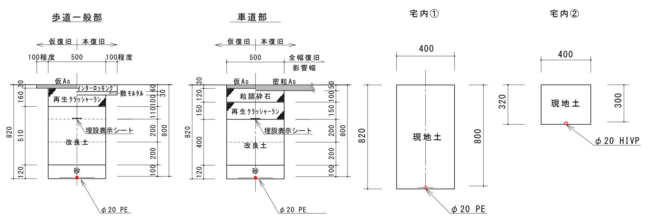
道路掘削復旧断面図 S=1/20
