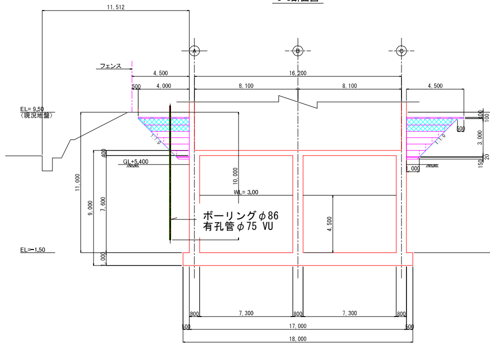
3-3断面図
