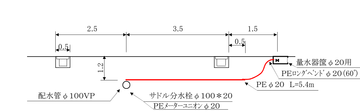
A-A断面図
