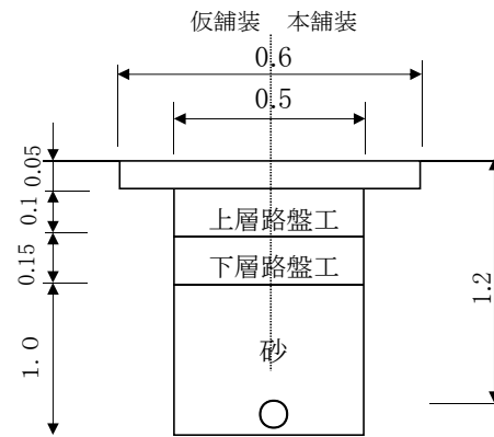
道路掘削復旧断面図
